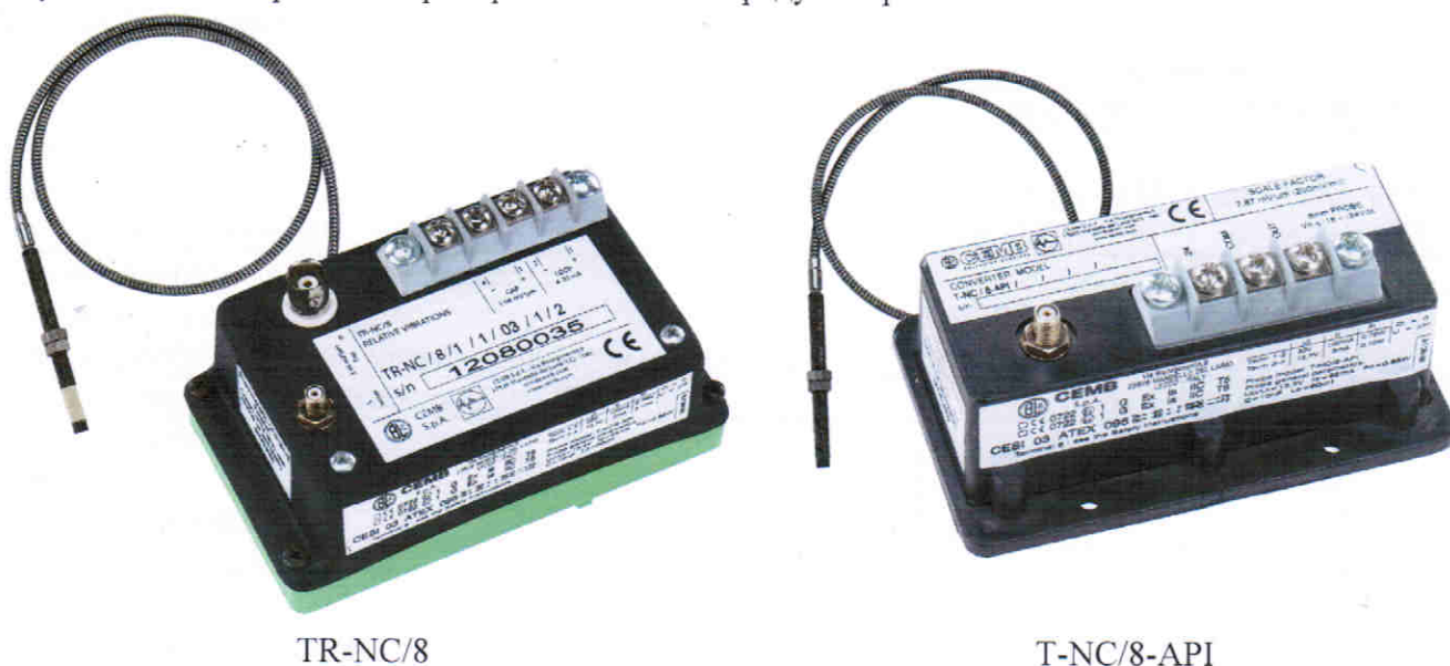
Рисунок 1 - Общий вид датчиков вихретоковых моделей TR-NC/8 и T-NC/8-API
